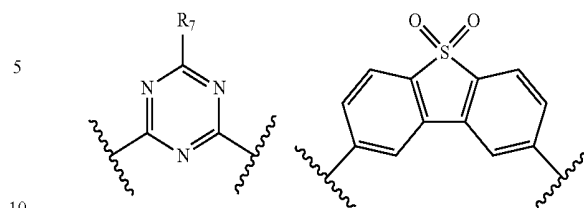
[Formula 5]
