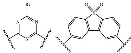
[Formula 5]
